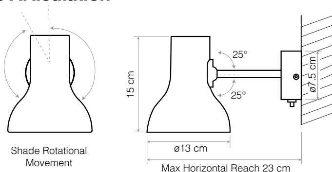
Type 75™ Mini Wall Light - Margaret Howell Edition
